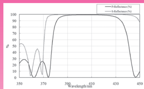
405nm Laser Mirror(45deg)
